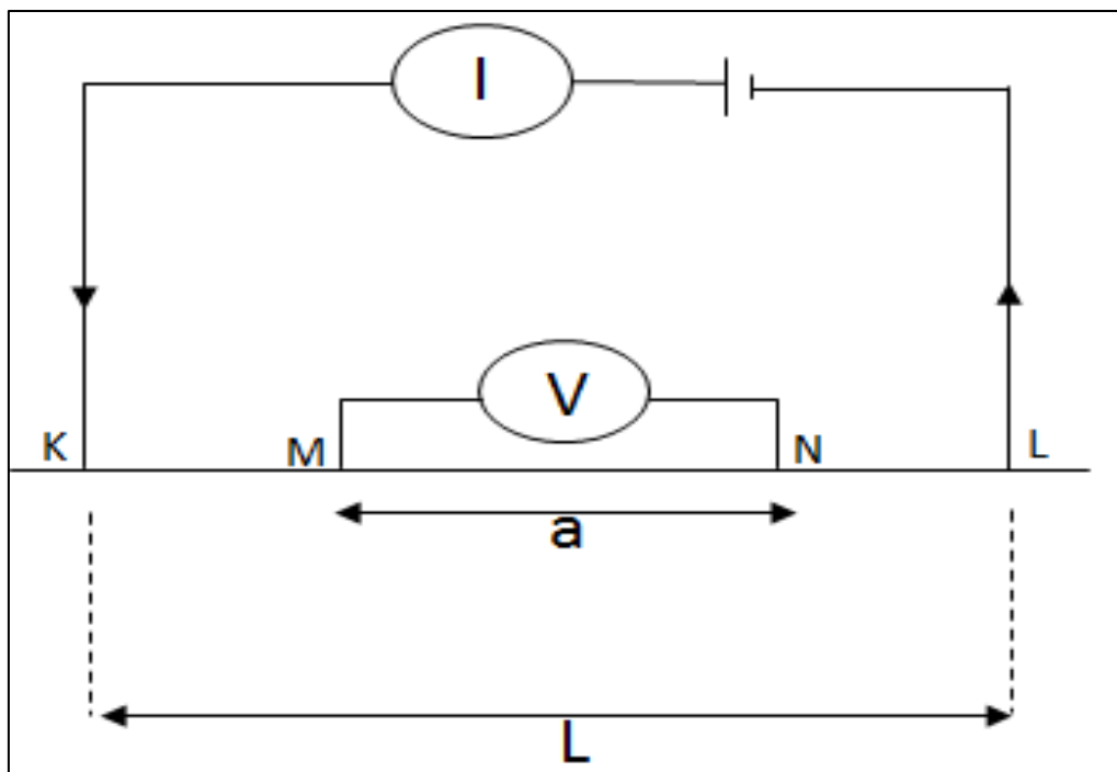
Figure-3. Schlumberger array method
